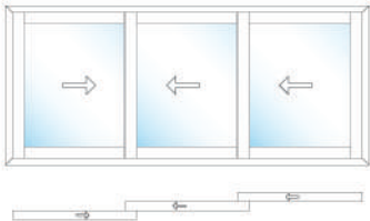
F2 90° Klasik Sürme 90° Classical Slide
