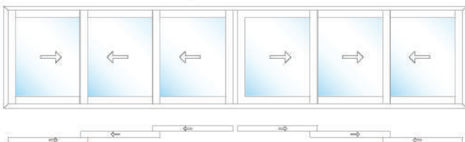
F2 90° Klasik Sürme 90° Classical Slide
