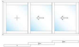
E4 90° Klasik Sürme 90° Classical Slide
