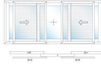
C2 90° Tek Ray Klasik Sürme 90° Monorail Classical Slide
