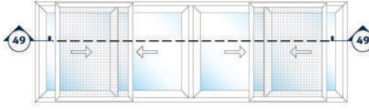
D1 45° Sineklik Klasik Sürme 45° Flyscreen Classical Slide
