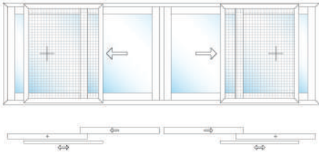
E3 90° Klasik Sürme 90° Classical Slide
