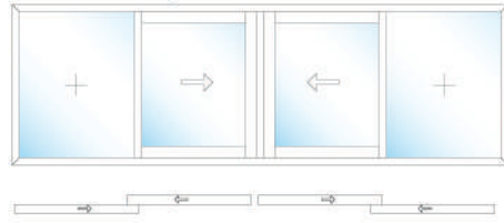
D3 90° Sineklik Klasik Sürme 90° Flyscreen Classical Slide
