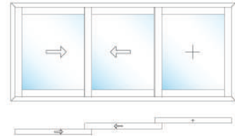
F3 90° Klasik Sürme 90° Classical Slide
