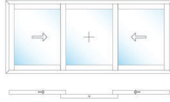
B5 90° Sineklik Klasik Sürme 90° Flyscreen Classical Slide
